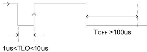
图4 一线脉冲时序图
