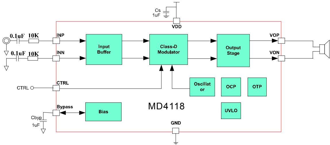
图2 MD4118原理框图
