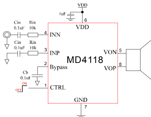
MD4118 典型应用电路
