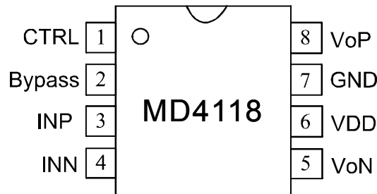
图1 ESOP8 装管脚分配图(top view)
