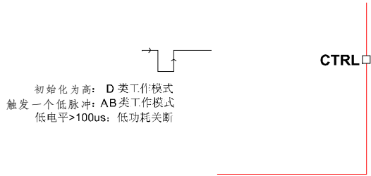
图3 MD 4118工作模式设置
